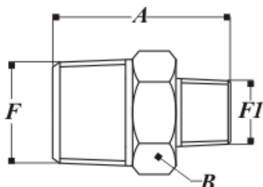
REDUCCION MACHO-MACHO
