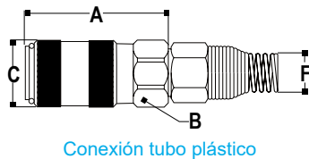
Conexión tubo plástico
